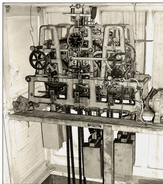
1. Asi dnes nejstarší pendlovky s napůl dřevěnými kolečky a vteřinovým kyvadlem (od Valtrů) 2. Přesné pendlovky z rychtářského stavení („Procházekovo“) – prosklenou skříňku již sežral červotoč. 3. Věžní hodiny „zezadu“ – prostřední závaží „pohání“ ručičky, pravé bití čtvrt-hodin, levé bití celých hodin
